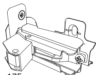
H5-1 - šarka 175 H5-2-bazeta 175
