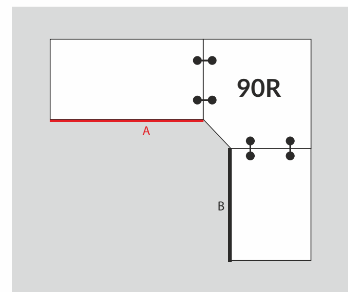
Typ pracovní desky L3 90R
