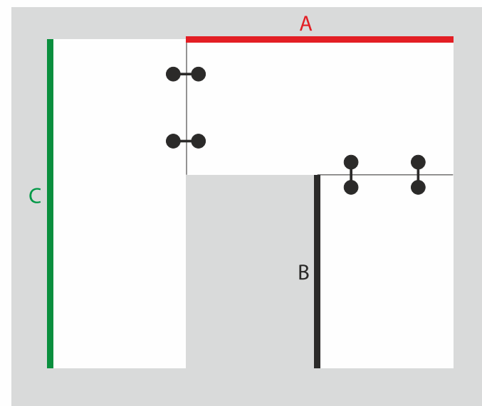
Typ spoje pracovní desky U2
