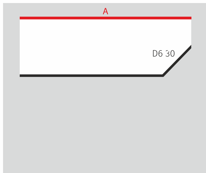
Typ spoje pracovní desky R2 levá
