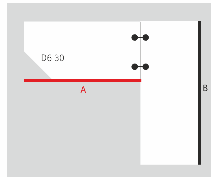
Typ spoje pracovní desky LR2
