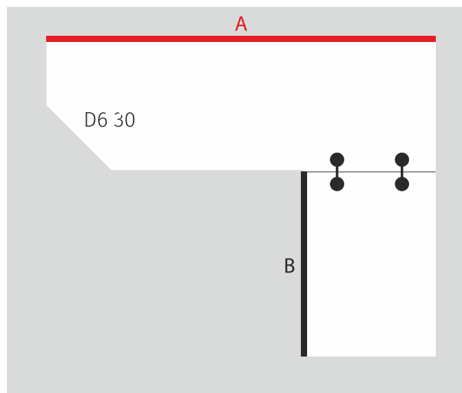
Typ spoje pracovní desky LR1
