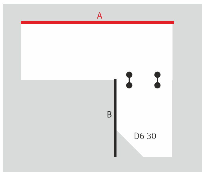
Typ spoje pracovní desky LR4
