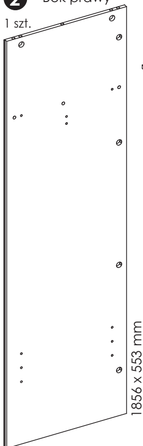
2 Bok prawy
